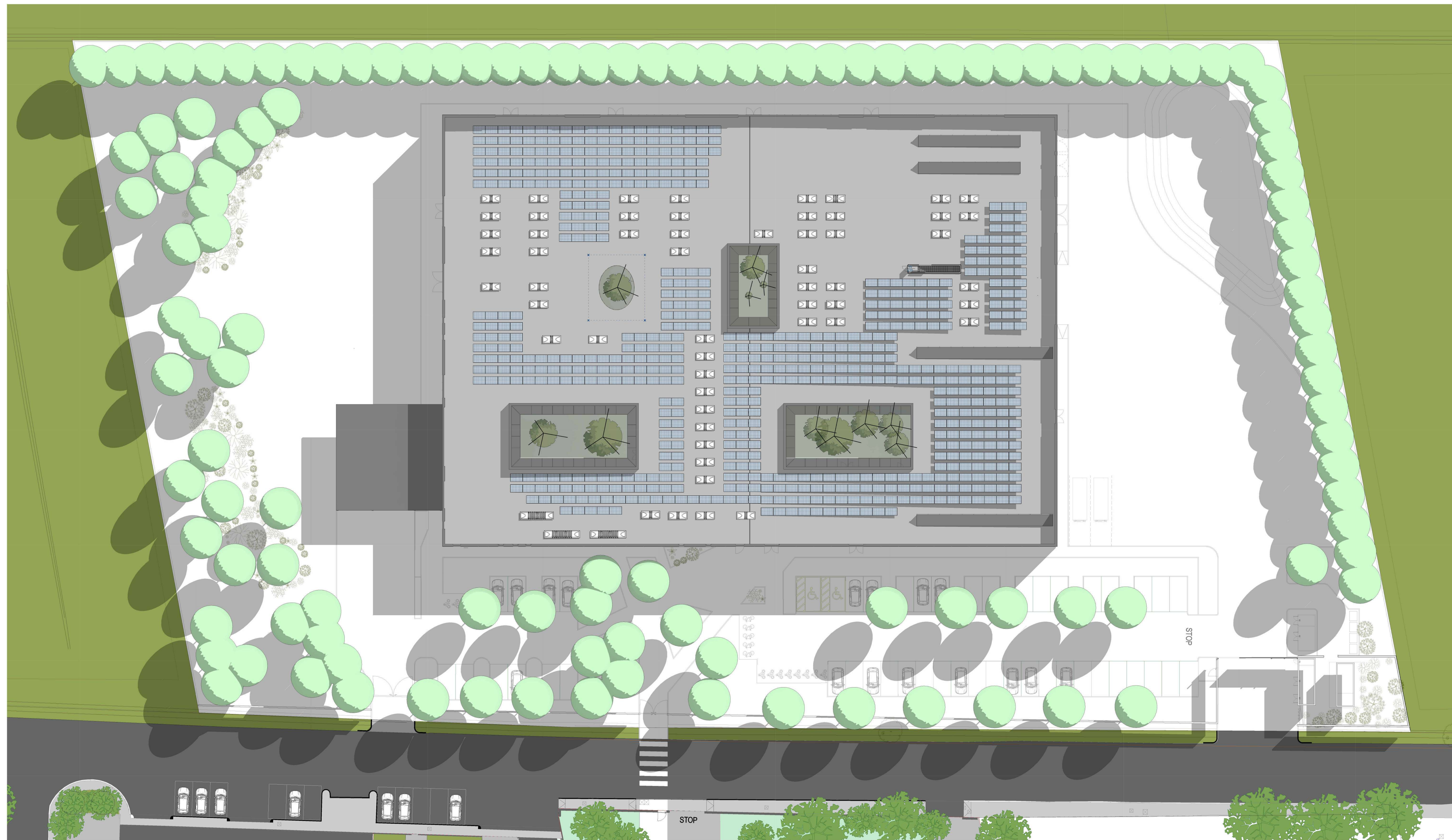
Planivolumetria Scale 1:200
