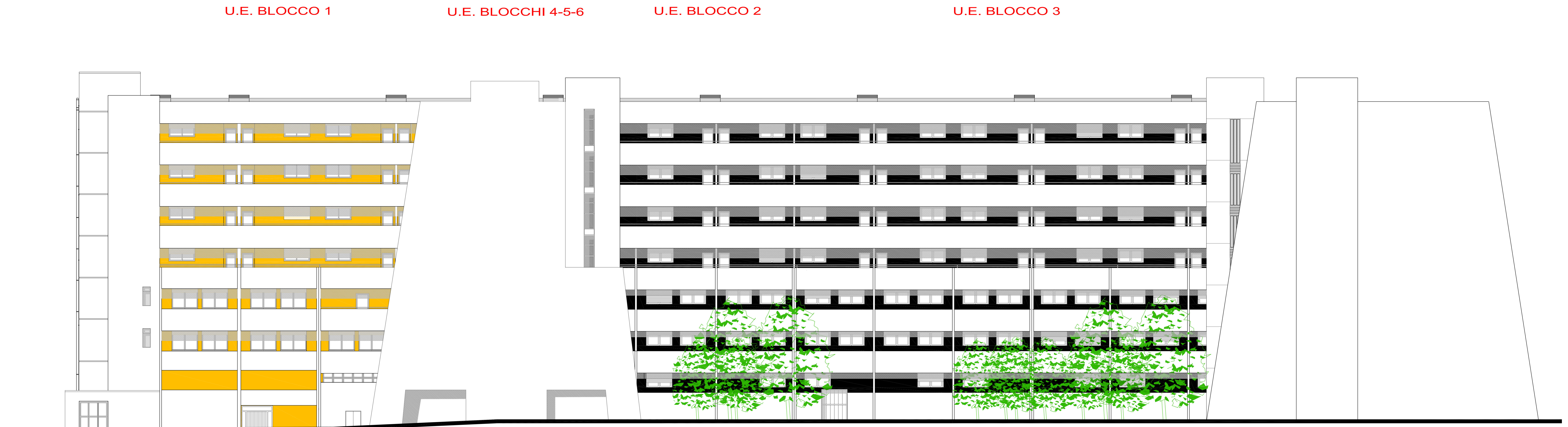
STATO DI FATTO - PROSPETTO SUD
