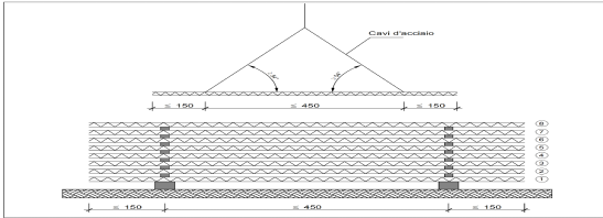
Figura 20.6 Esempio di stoccaggio di travetti tralicciati
