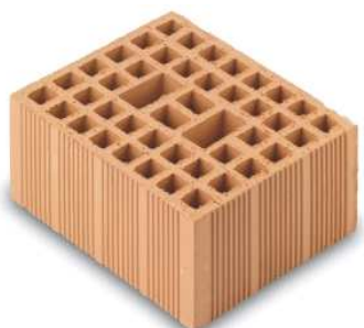
Figura 18.4 Esempi di blocchi forati 45% < \phi \leq 55% in laterizio per murature portanti
