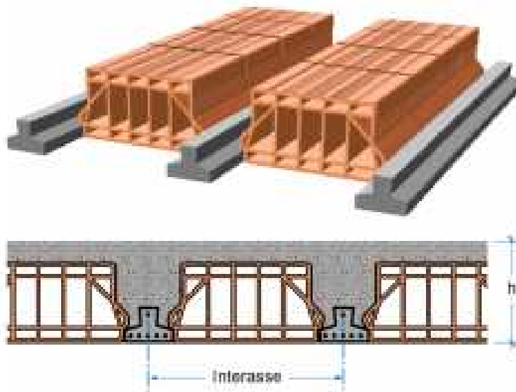
Figura 20.3 Esempio di solaio in cemento armato a travetti in cemento armato e blocchi interposti (fonte: Laterificio Pugliese s.p.a.)
