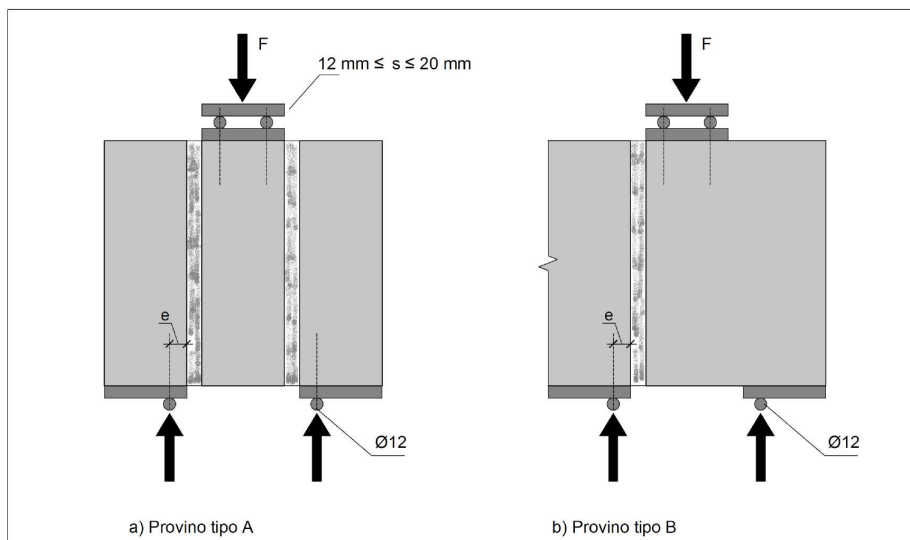
Figura 18.6 Carico di prova per la determinazione sperimentale della resistenza a taglio (modificata UNI EN 1052-3)
