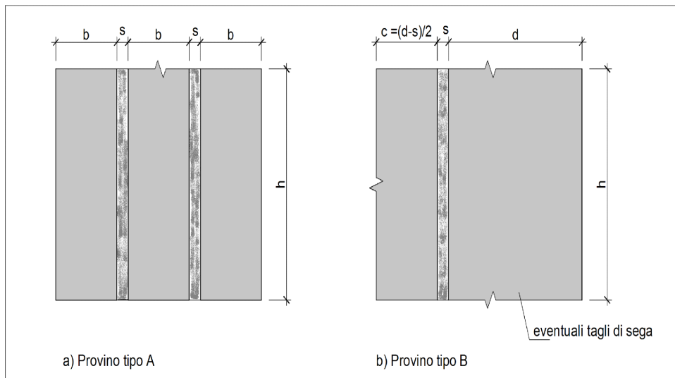
Figura 18.5 Dimensioni dei provini di muratura per prova di determinazione sperimentale della resistenza a taglio
