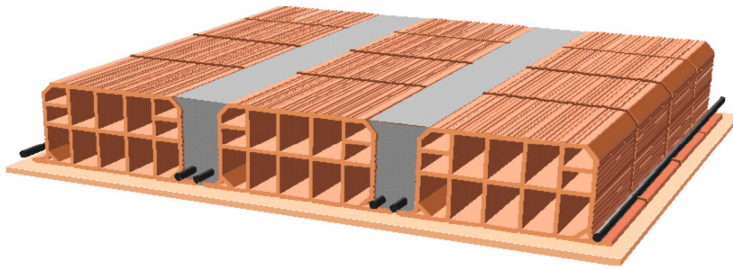
Figura 20.1 Esempio di solaio in cemento armato gettato in opera (fonte: Laterificio Pugliese s.p.a.)
