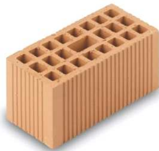
Figura 18.2 Esempio di mattone semipieno 15\% < \phi \leq 45\% in laterizio per murature portanti (fonte: www.fornacetrezzo.it )
