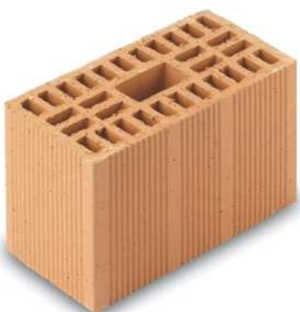
Figura 18.3 Esempi di blocchi semipieni 15% < \phi \leq 45% in laterizio per murature portanti
