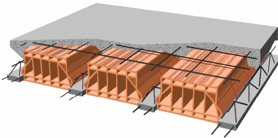
Figura 20.2 Esempio di solaio in cemento armato a travetti tralicciati e blocchi interposti (fonte: Laterificio Pugliese s.p.a.)
